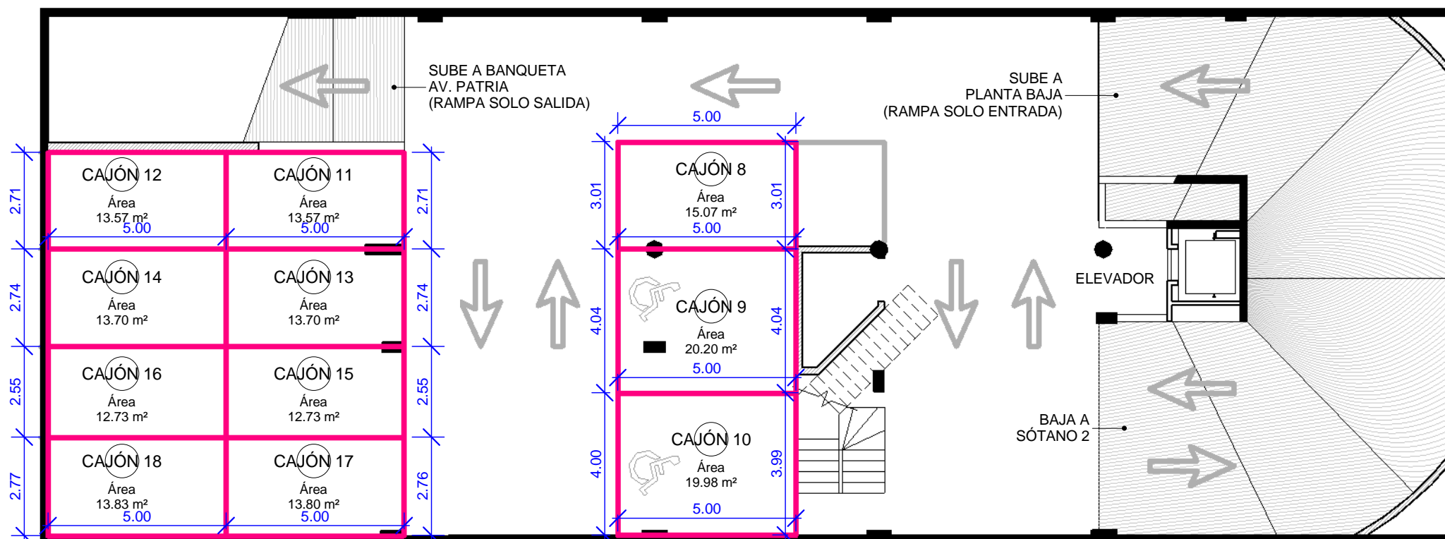
2 SÓTANO 1
