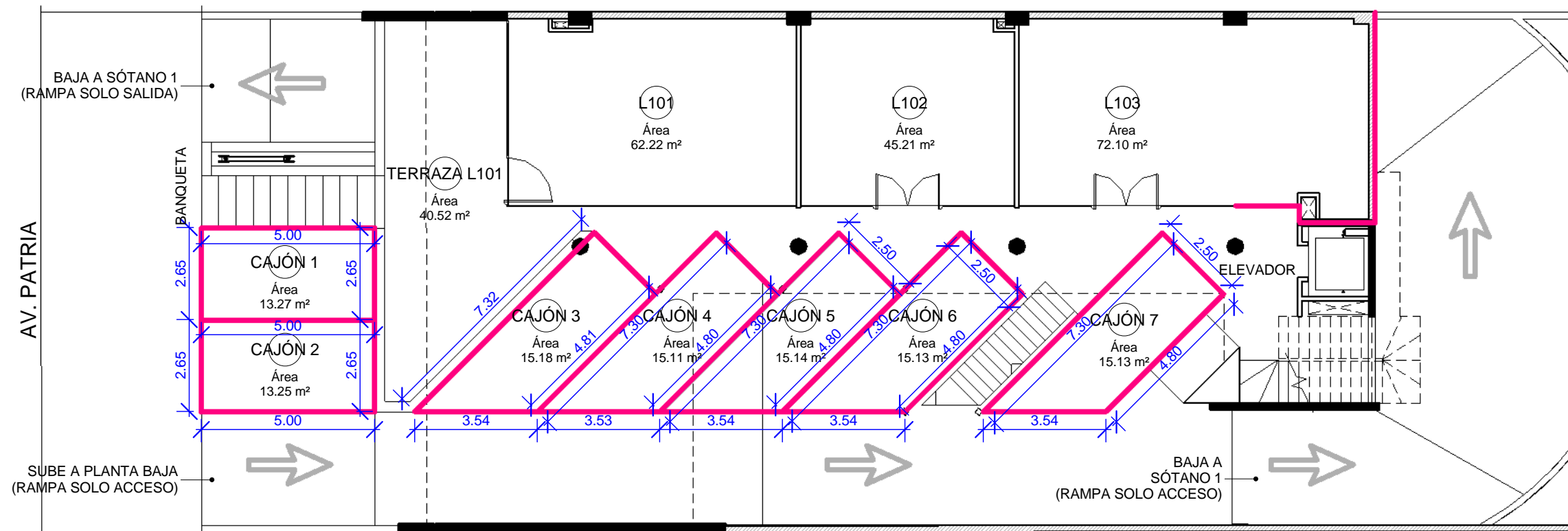
1 PLANTA BAJA
